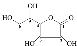
RYCINA 2. Wzór strukturalny kwasu L-askorbinowego
